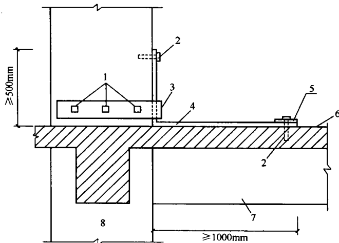
图 10.9.3-3 柱中部加贴 L 形钢板及 U 形钢箍板的锚固构造示例
