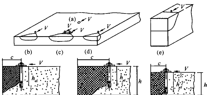
图 16.3.1-2 混凝土边缘呈楔形受剪破坏
