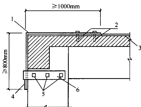
(a) 柱顶加贴L形钢板的构造
