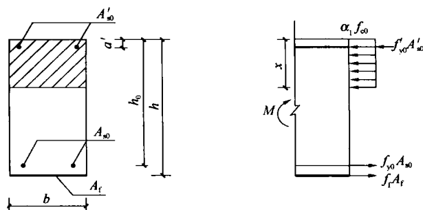
图 11.2.3 矩形截面正截面受弯承载力计算
