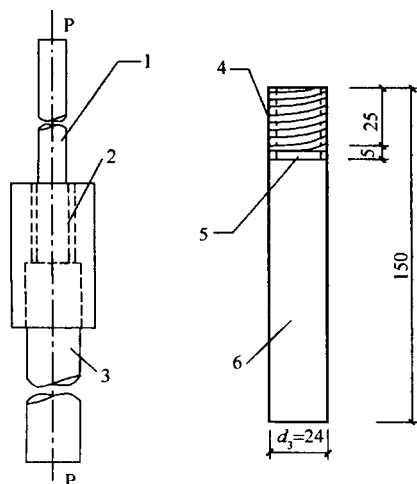
图 C.6.1 试件安装钢螺杆
