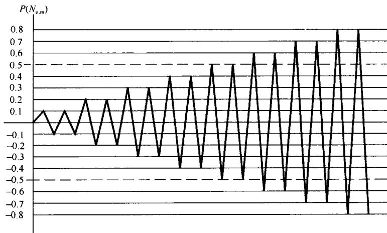
图 D. 5. 4 抗震性能检验加载制度
