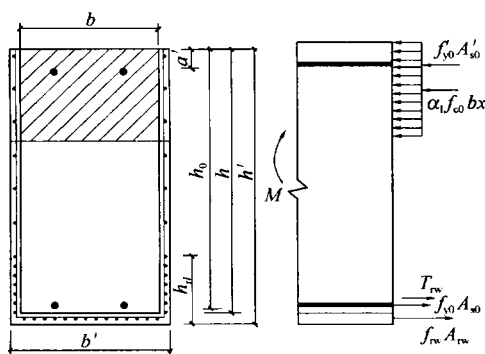
(a) 围套式外加固原计算图
