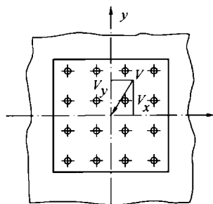
图 F. 2. 2 受剪力作用
