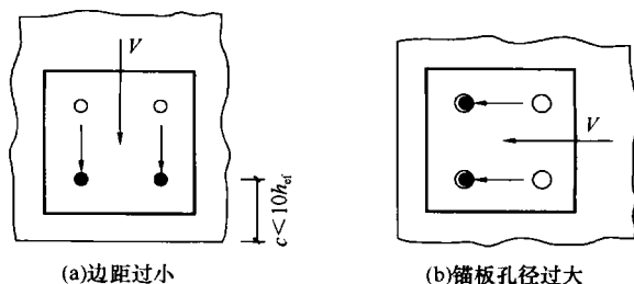
图 F.2.1-2 锚栓处于不利情况下受剪
