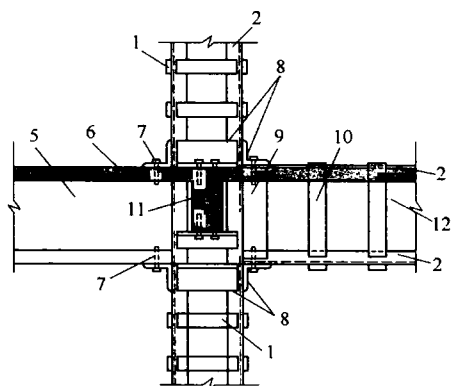
(b)外粘型钢梁、柱节点构造
