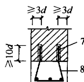
(c) 植筋埋设 U 形箍构造
