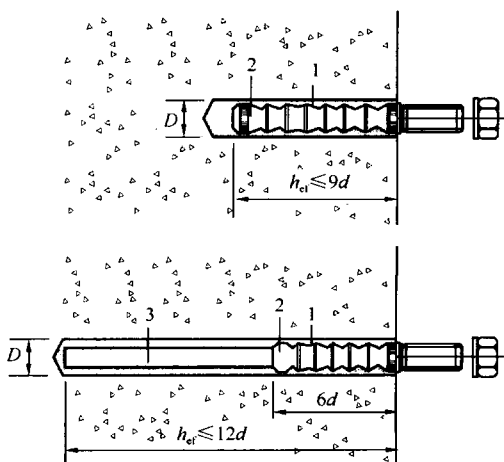
图 16.1.3-2 特殊倒锥形胶粘型锚栓
