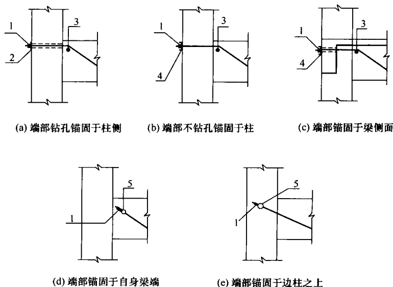
图 7.5.3 端部锚固构造示意图
