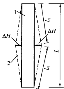
图 7.4.1 预应力撑杆横向张拉量计算图
