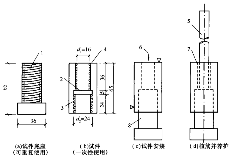
图 C.3.1 标准试件的形式与尺寸 (mm)
