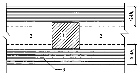
图 10.9.3-1 绕过柱位粘贴纤维复合材
