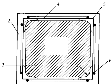
图 8.1.3 外粘型钢加固
