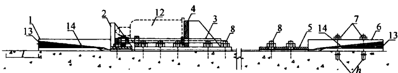
图 11.1.10-2 张拉前锚具纵向剖面示意图
