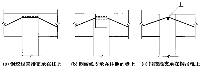
图 7.5.2 中间连续节点构造方法
