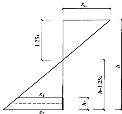
图 1 应变平截面假定图
