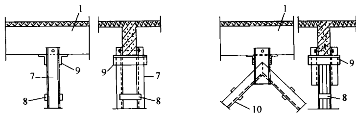
(b) 型钢套筒干式连接
