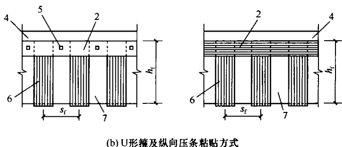
图 10.3.1 纤维复合材料抗剪箍及其粘贴方式
