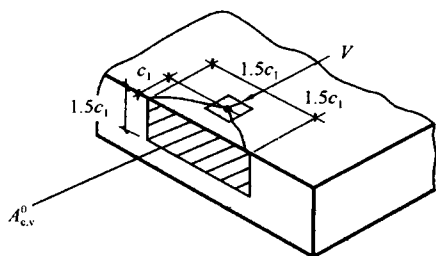
图 16.3.8 近构件边缘的单锚受剪混凝土楔形投影面积
