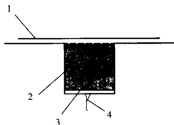
图 3 裂缝处开 U 形沟 槽充填修补材料
