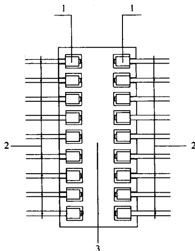
图 13.4.4 主绳连接锚固构造示意图
