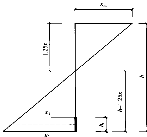
图 2 应变平截面假定图
