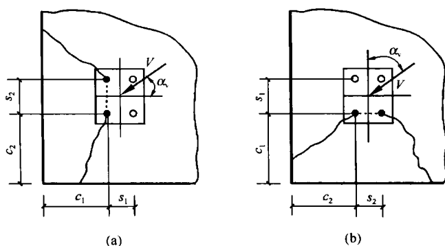
图 16.3.11 剪力作用下的角部群锚
