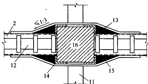
(c)外粘型钢梁、柱节点构造
