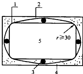
图 14.3.1 绕丝构造示意图
