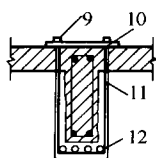
(d) 环形箍筋或加锚式箍筋构造
