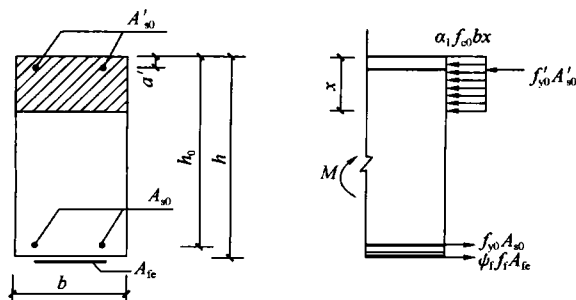
图 10.2.3 矩形截面构件正截面受弯承载力计算
