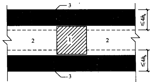
图 9.6.4-1 绕过柱位粘贴钢板
