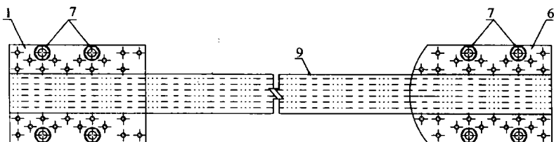
图 11.1.10-3 张拉完成锚具平面示意图
