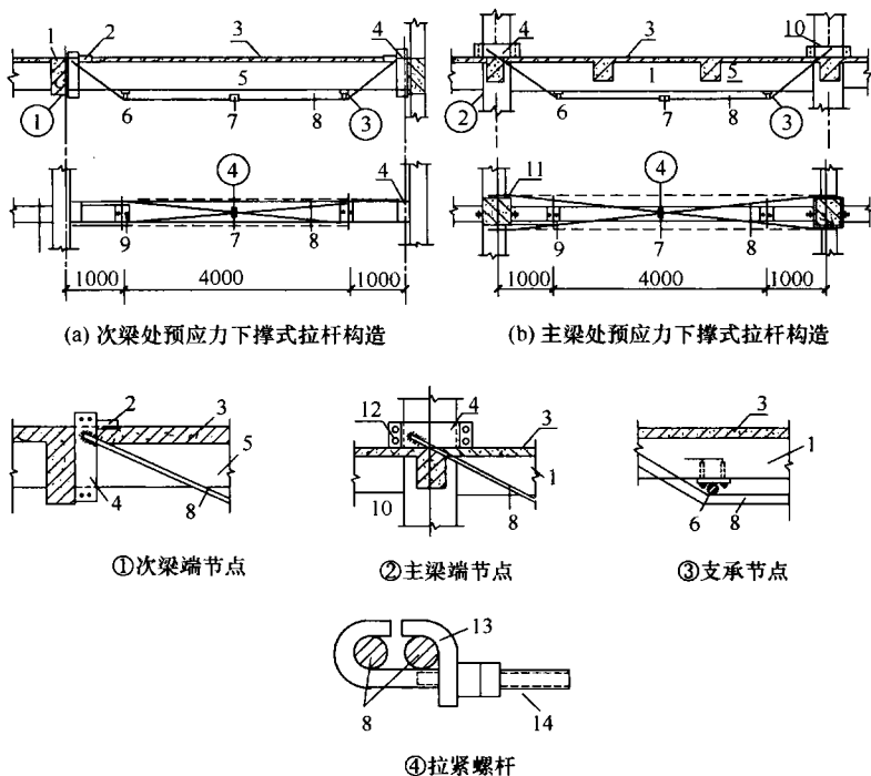
图 7.6.1 预应力下撑式拉杆构造
