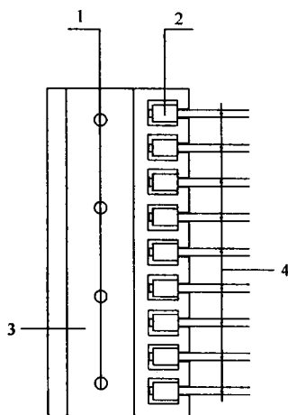
图 13.4.1-2 采用固定结紧固钢丝绳的 端头锚固构造
