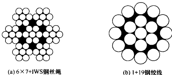
图 13.4.1-1 钢丝绳的结构形式
