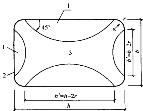
图 10.4.4 环向围束内矩形截面有效约束面积
