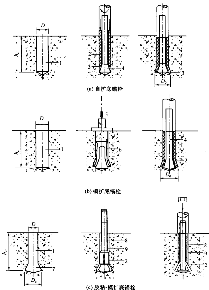
图 16.1.3-1 后扩底锚栓
