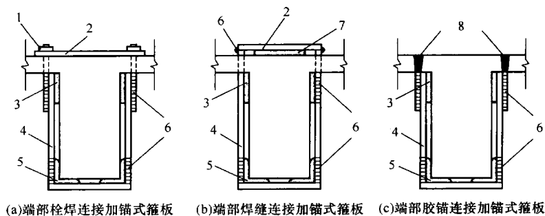
图 8.3.1 加锚式箍板
