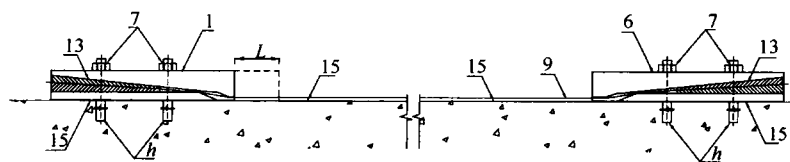
图 11.1.10-4 张拉完成锚具纵向剖面示意图
