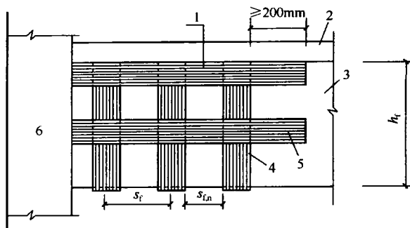
图 10.9.6 纵向腰压带
