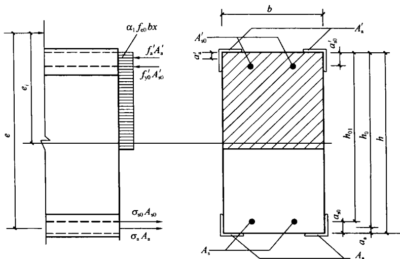
图 8.2.2 外粘型钢加固偏心受压柱的截面计算简图
