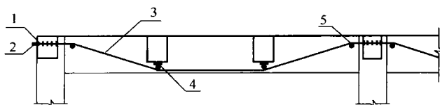
(a) 钢绞线布置形式1
