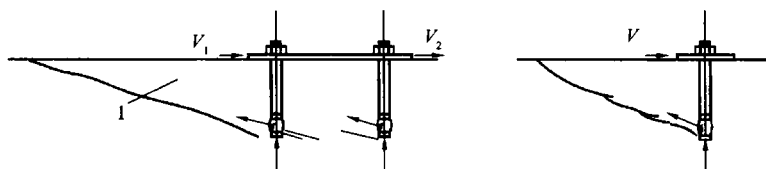
图 16.3.1-3 混凝土剪撬破坏
