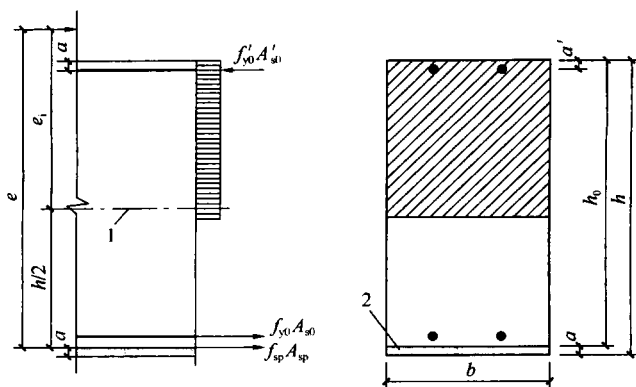
图 9.4.2 矩形截面大偏心受压构件粘钢加固承载力计算
