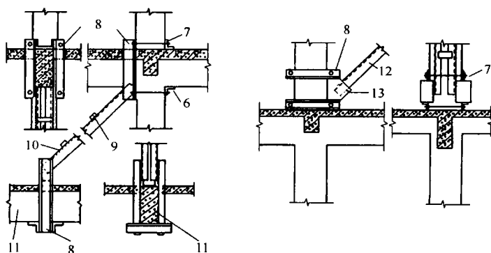
(b) 型钢套箍干式连接
