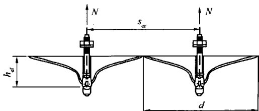
图 16.3.1-1 混凝土呈锥形受拉破坏
