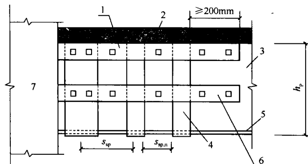
图 9.6.6 纵向腰间钢压条
