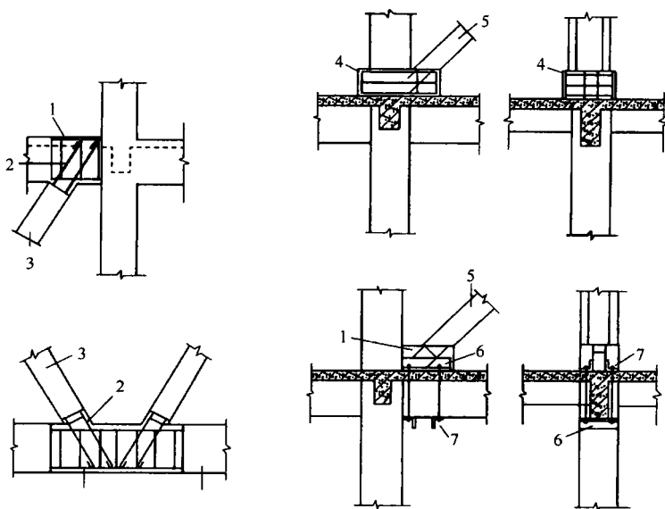
(a) 钢筋混凝土围套湿式连接
