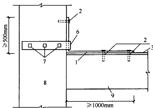
(b) 柱中部加贴L形钢板的构造
