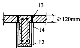
(e) 环形箍筋或加锚式箍筋构造
