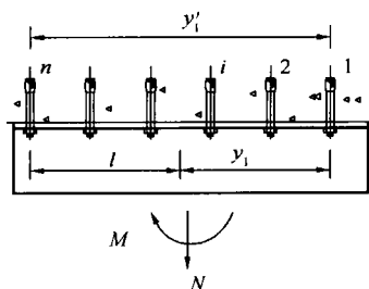
图 F.1.1-2 拉力和弯矩共同作用
