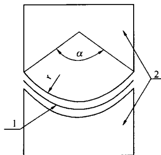
图 11.3.5-2 圆齿齿纹锚具单齿示意图
