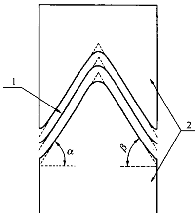
图 11.3.3-2 尖齿齿纹锚具单齿示意图
