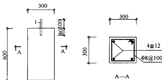
图 D.3.1 种有螺杆的试件 (单位 mm)
