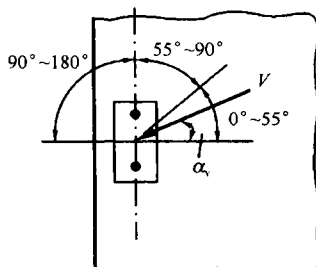
图 16.3.7 剪切角 \alpha_v
