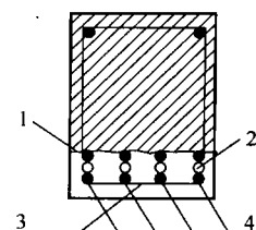
(a) 短筋焊接连接构造
