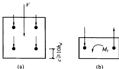
图 F.2.1-1 锚栓均匀受剪
