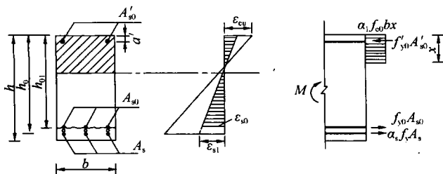
图 5.2.3 矩形截面受弯构件正截面加固计算简图
