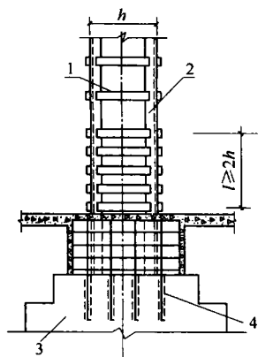
(a)外粘型钢柱、基础节点构造
