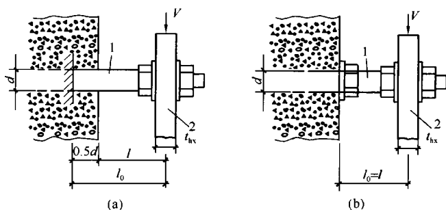
图 16.2.4 锚栓杠杆臂计算长度的确定
