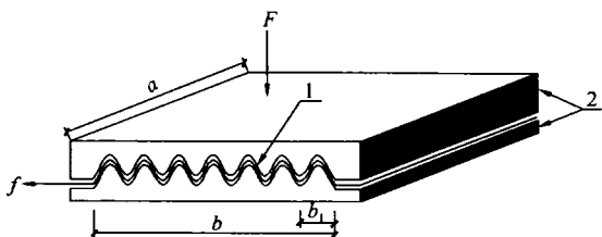
图 11.3.3-1 尖齿齿纹锚具示意图
