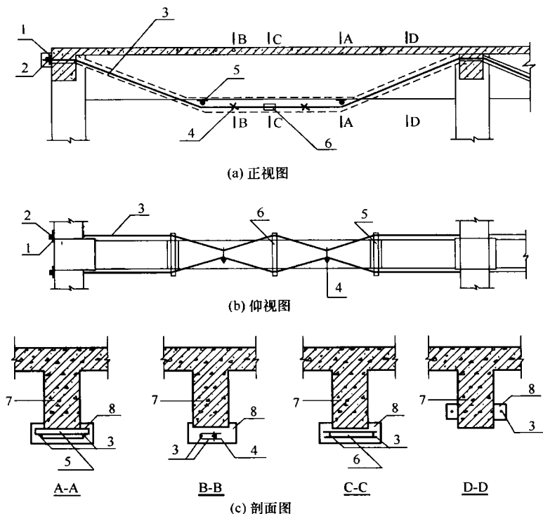
图 7.5.5 采用横向张拉法施加预应力
