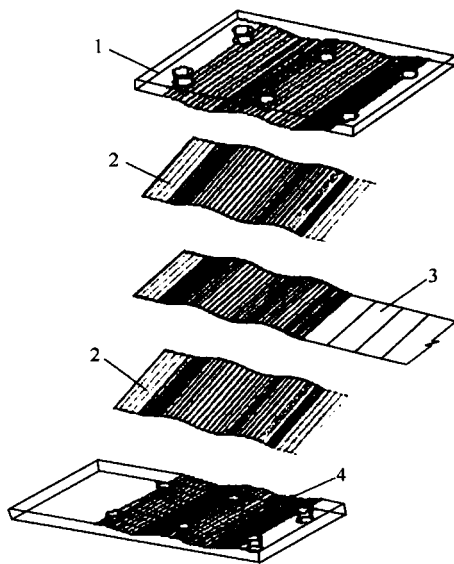
图 11.3.12 锚具内加贴的碳纤维织物垫层
