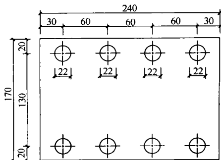
图 11.3.2-2 平板锚具盖板和底板平面
