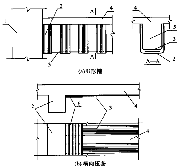
图 10.9.2 梁、板粘贴纤维复合材端部锚固措施
