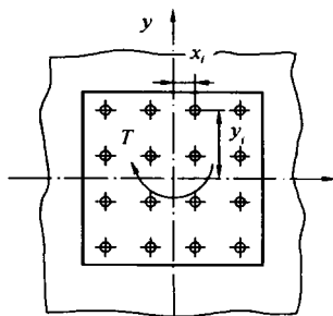
图 F. 2. 3 受扭矩作用
