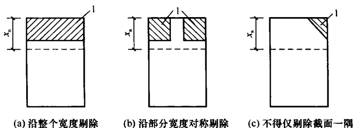
图 6.3.3 梁置换混凝土的剔除部位
