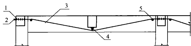
(b) 钢绞线布置形式2
