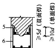
(b) 设置 U 形箍筋构造
