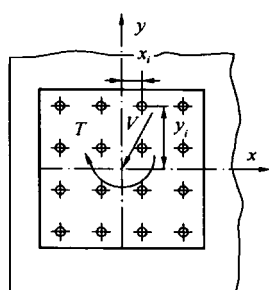
图 F. 2. 4 剪力与扭矩共同作用
